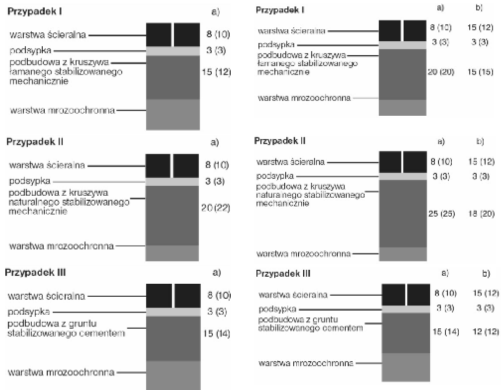
2.3. Konstrukcja nawierzchni dla kategorii ruchu R_2 – grubość warstwy w [cm]
