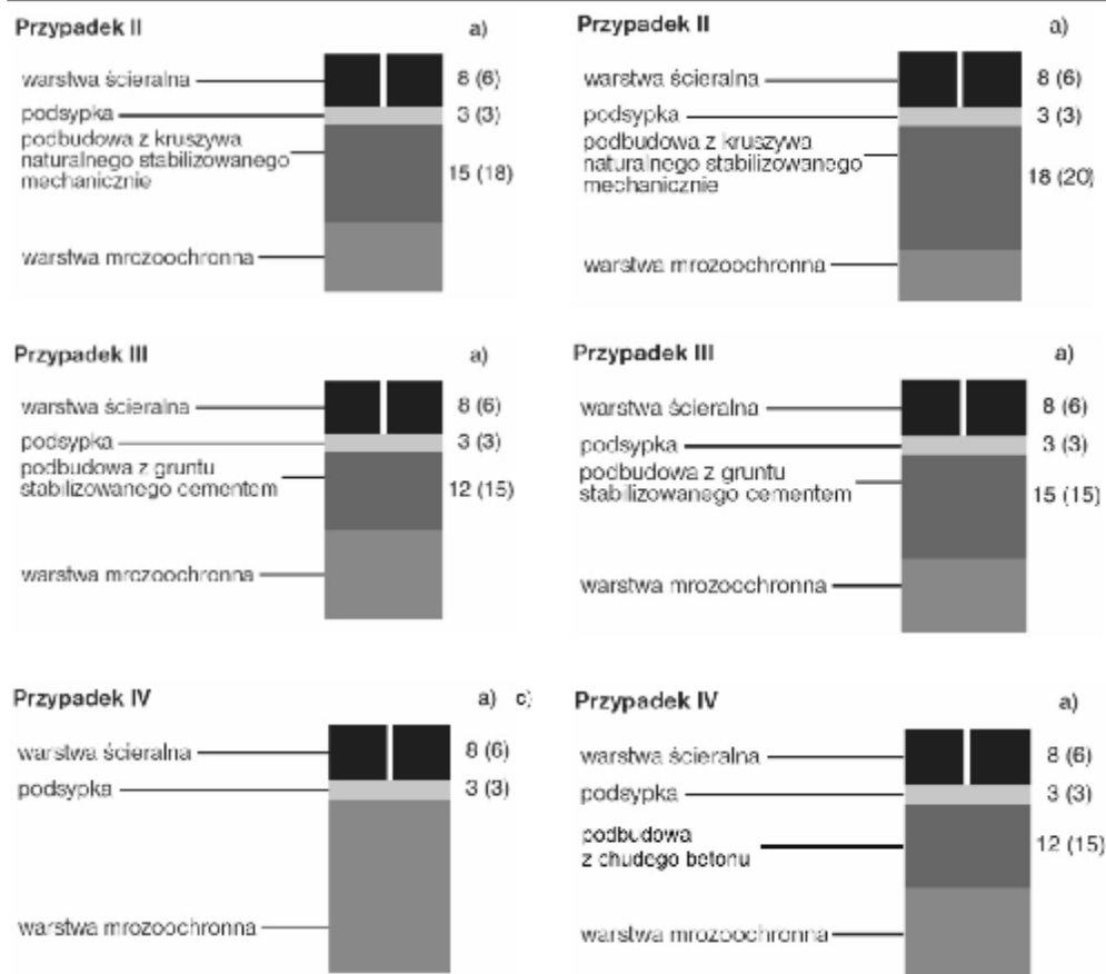
2.3. Konstrukcja nawierzchni dla kategorii ruchu R_2 – grubość warstwy w [cm]
